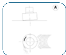
Taglio radiale Radial grinding 径向磨削
