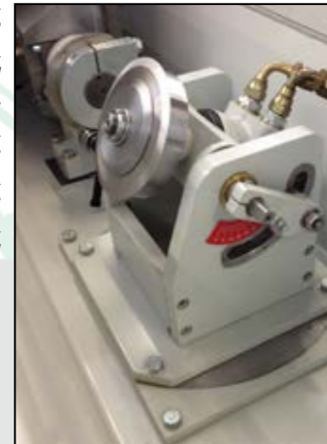
Affilatura disco circolare - angolo di taglio
