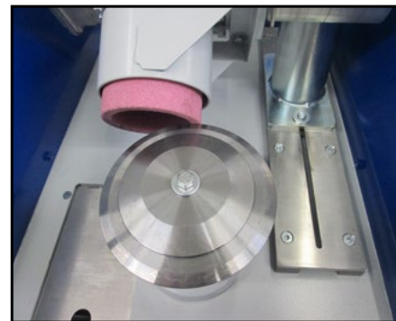
Mola Ø100 mm Grinding wheel Ø100 mm Шлифкруг Ø100 мм
