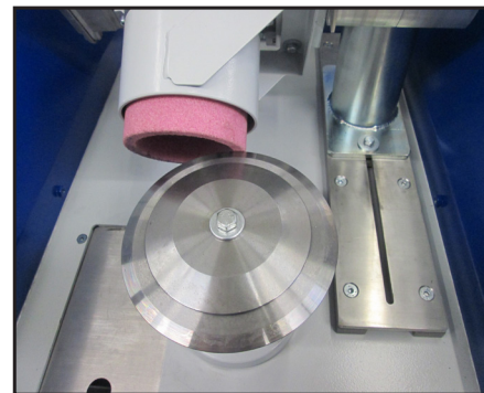
Mola Ø100 mm Grinding wheel Ø100 mm 砂轮直径100毫米
