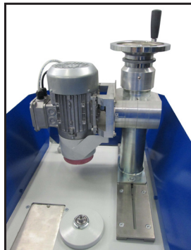
Mandrino con motore 0,37 Kw Motor spindle 0,37 kW 电机主轴 0.37千瓦
