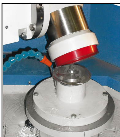
Flangia per tavola rotante Flange for standard rotating table Flansch für Standard-Drehtisch
