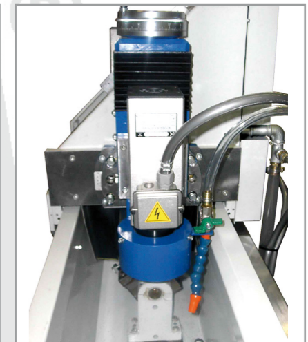
Testa di superfinitura 1,1 kW
