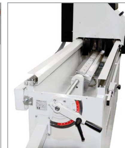
Leva rotazione del piano elettromagnetico 0°/90°
